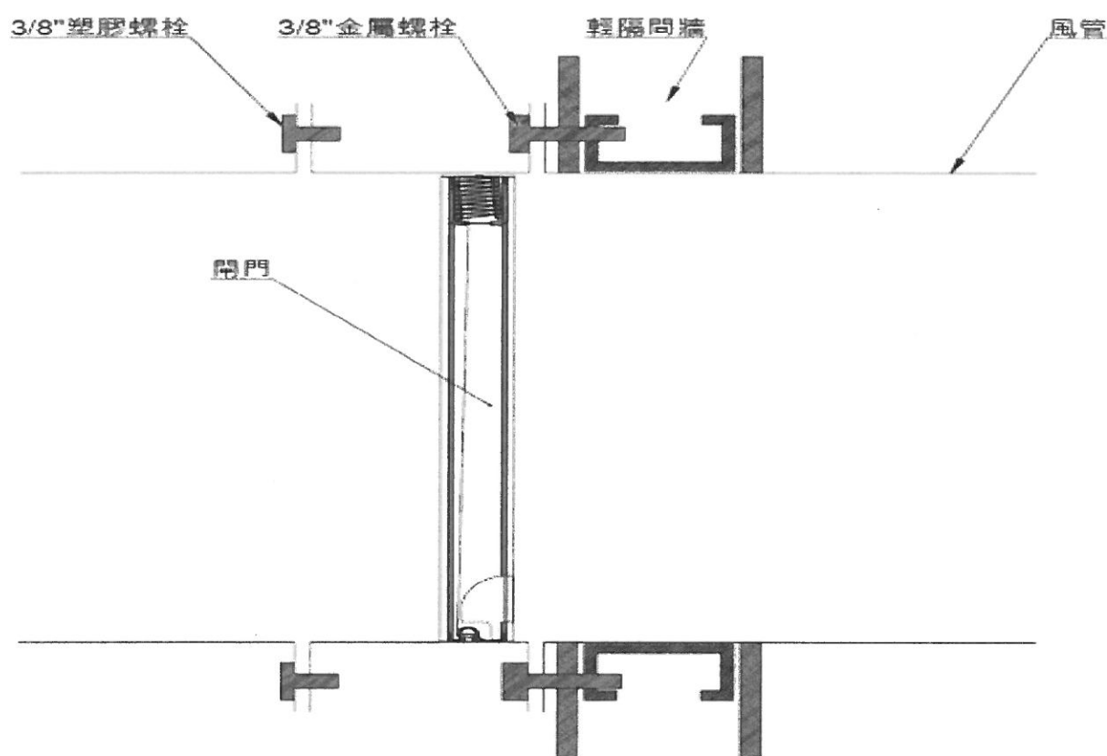
圖一、掛牆剖面結合圖(示意圖)
